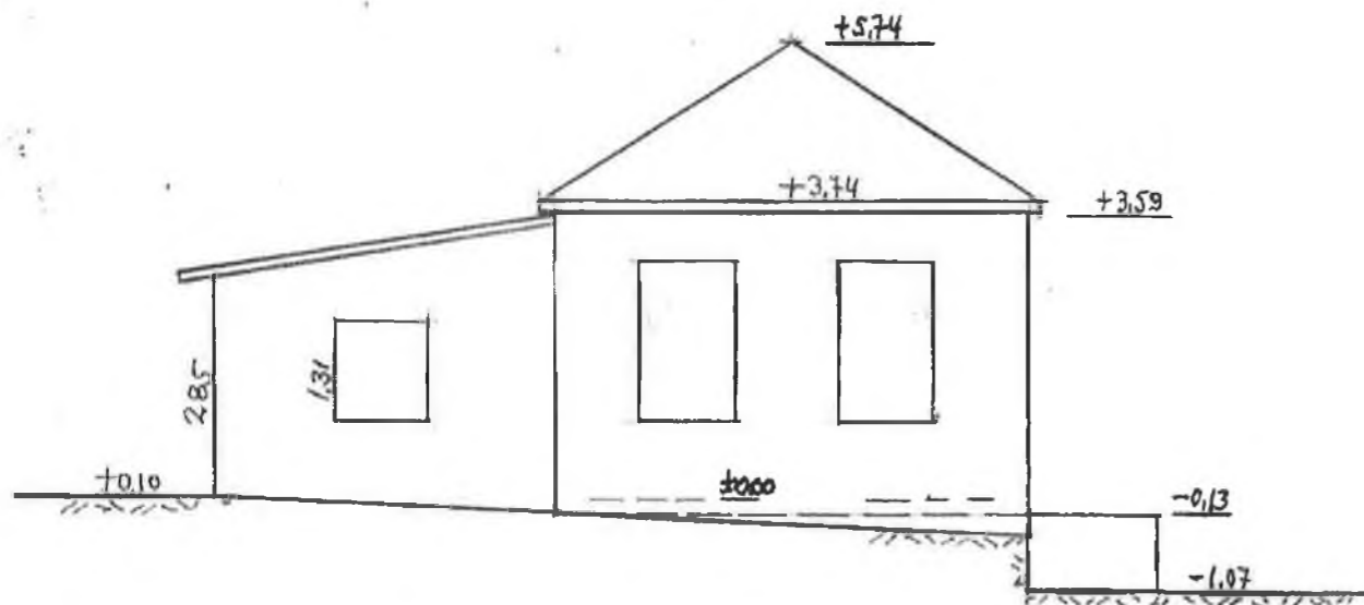
ΛΟΓΟΓΡΑΦΙΚΟ ΜΟΥΣΕΙΟ | ΔΗΜΟΤΙΚΟ ΣΧΟΛΕΙΟ | ΔΥΤΙΚΗ ΟΨΗ 1:100
