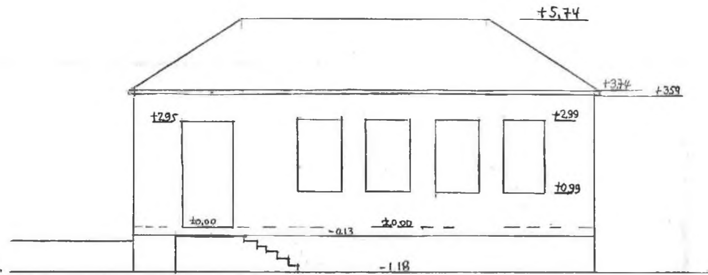
ΝΟΤΙΑ ΟΨΗ 1:100
