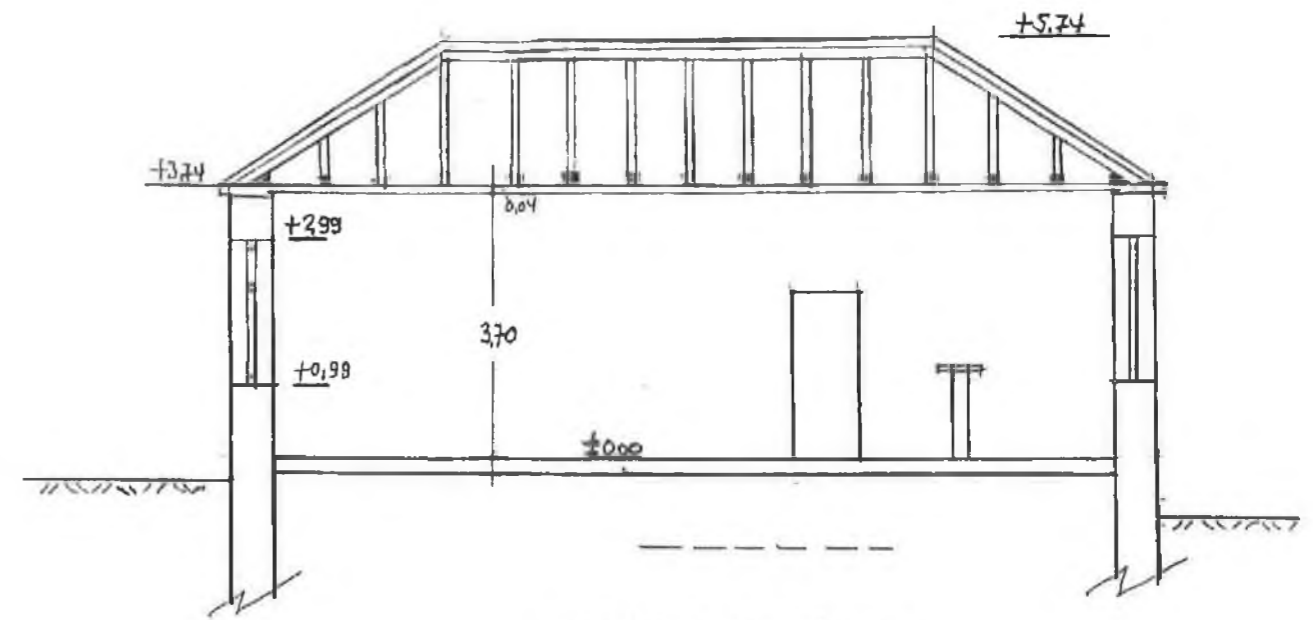
ΤΟΜΗ Α-Α 1:100
