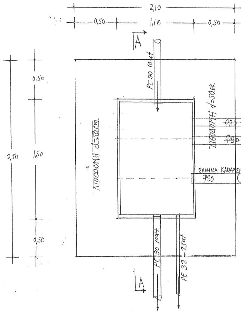
ΚΑΤΟΧΗ ΦΡΕΑΤΙΟΥ 1:20
