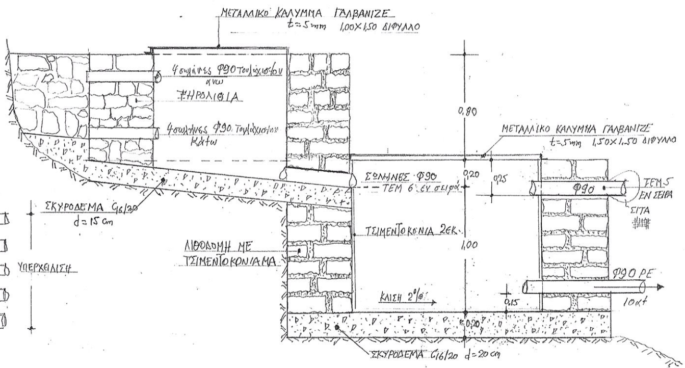
ΤΟΜΗ Α-Α 1:20
