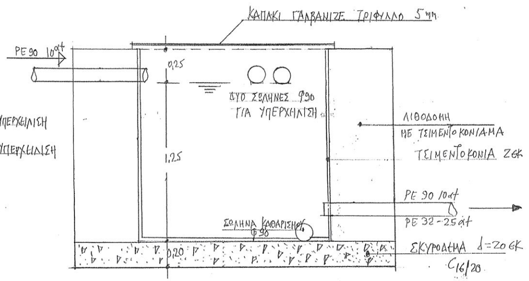
ΤΟΜΗ Α-Α 1:20
