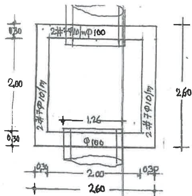
ΚΑΤΩΨΗ ΦΡΕΑΤΙΟΥ 1:50
