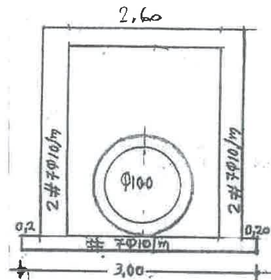
ΤΟΜΗ ΦΡΕΑΤΙΟΥ ΚΑΘ' ΥΨΟΣ
