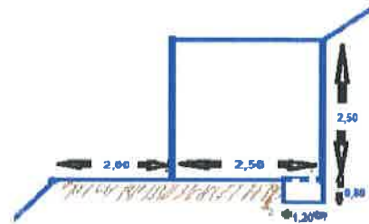
ΔΙΑΤΟΜΗ Δ,Ε
